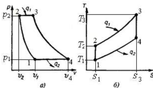
Рисунок 1.4 Цикл газотурбинной установки: а — в pV -координатах; б — в Ts -координатах
