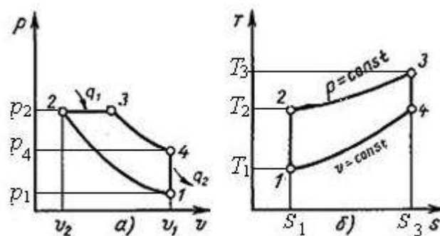
Рисунок 1.2. Цикл ДВС с изобарным подводом теплоты: a — в pV -координатах; б — в Ts -координатах
